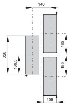
Schalttafelausschnitt / Panel aperture
